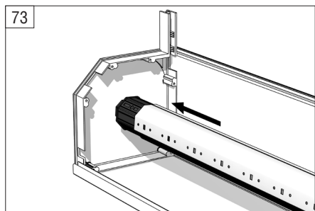
73. Выдвиньте универсальную капсулу из вала, до упора в крышку.
