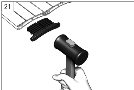
Установите боковые замки в ламели (тип замка SLE45, SLE55).
