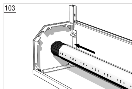
103 Выдвиньте универсальную капсулу из вала, до упора в крышку.
