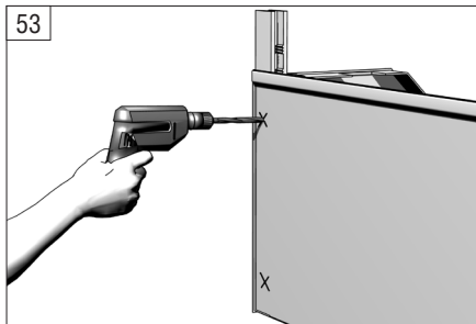
53 Просверлите отверстия в задней части короба под заклепки \varnothing 4 мм.
