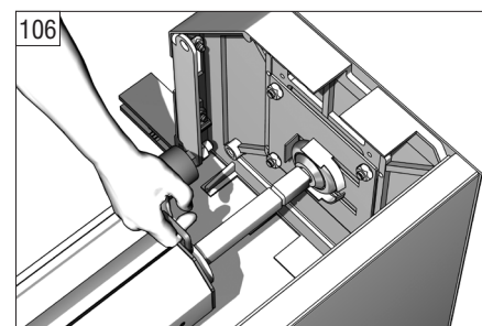
106 В случае с капсулой КРУ70, КРУ60 выдвиньте шток капсулы до упора в подшипник суппорта. Затяните фиксирующие винты. Внимание! Шток должен быть выдвинут на расстояние от края вала до боковой крышки не более 50 мм.
