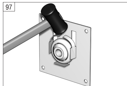
97 Загните пластины на суппорте BS42 для закрепления подшипника.
